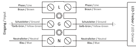
Elektrischer Anschluss / Electrical connection 90-305V AC, 50/60 Hz
